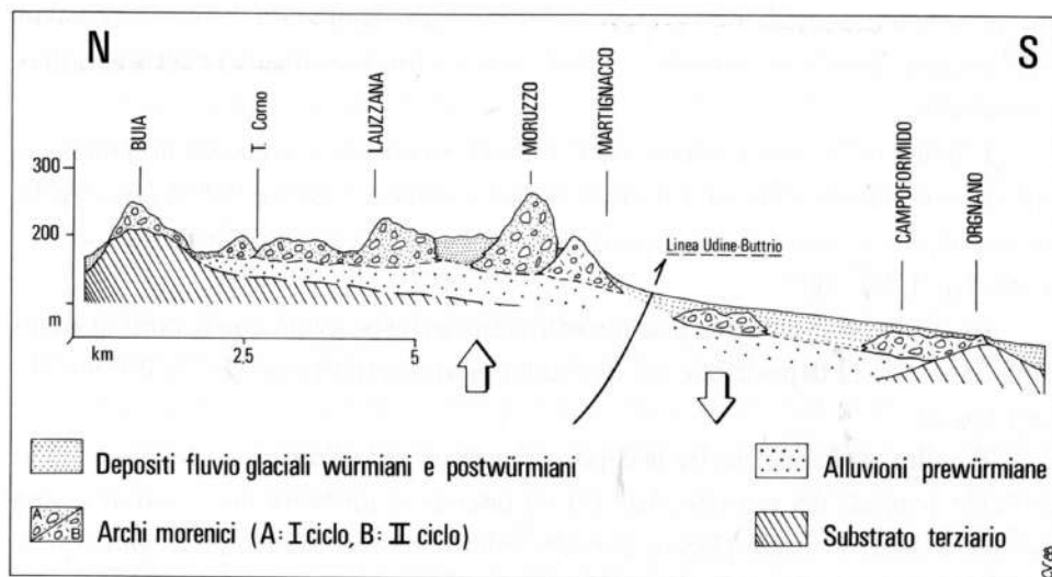
Fig. 3 - Sezione geologica lungo l'anfiteatro morenico affiorante e sepolto dell'alta pianura friulana. Da rimarcare il rigetto di età pleisto-olocenica operato dalla Linea Udine-Buttrio, valutabile in una trentina di metri e particolarmente evidente lungo questa sezione.
