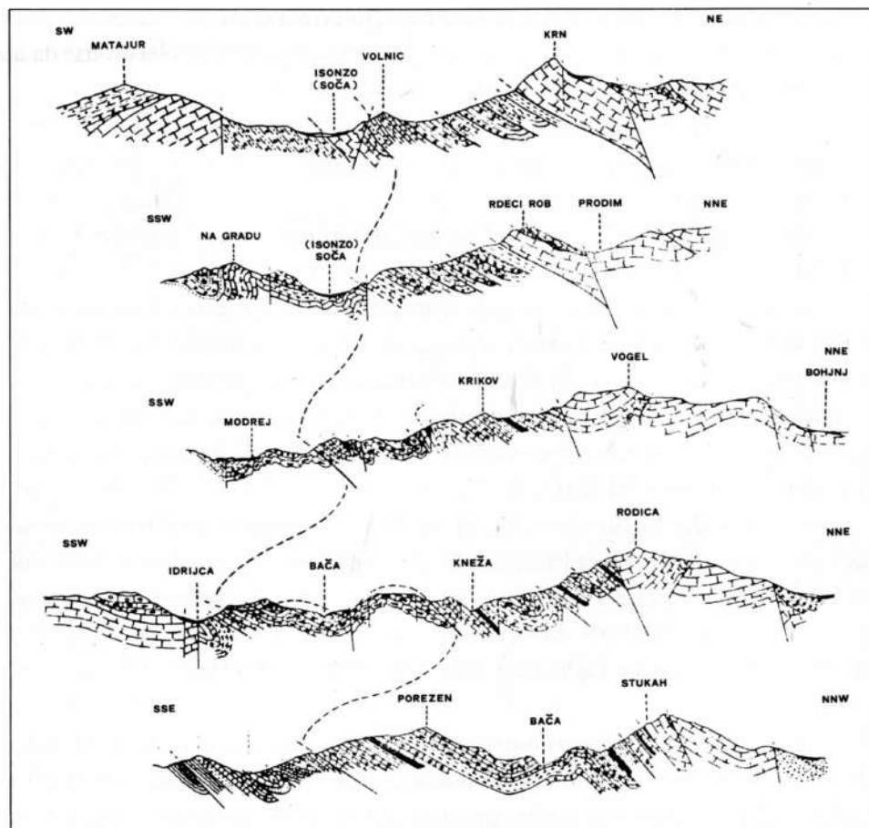
Fig. 6 - Sezioni geologiche dei monti di Tolmino (da Cousin, 1981). L'allineamento Krn - Peski - Vogel - Rodica - Stukah è caratterizzato da strutture di tipo transpressivo (strutture a fiore).
