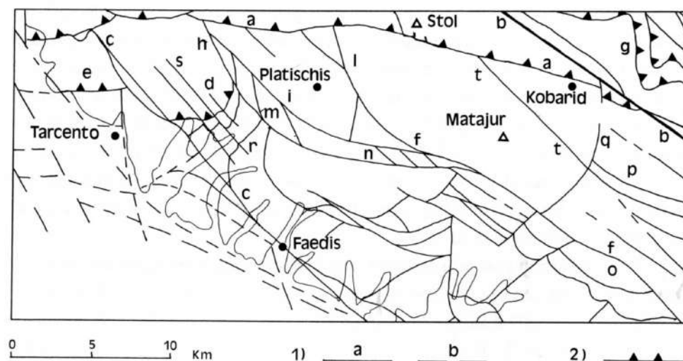
Fig. 1 - Schema tettonico delle Prealpi Giulie meridionali. 1. Faglie: a) certe; b) presunte o sepolte. 2. Sovrascorrimenti.
