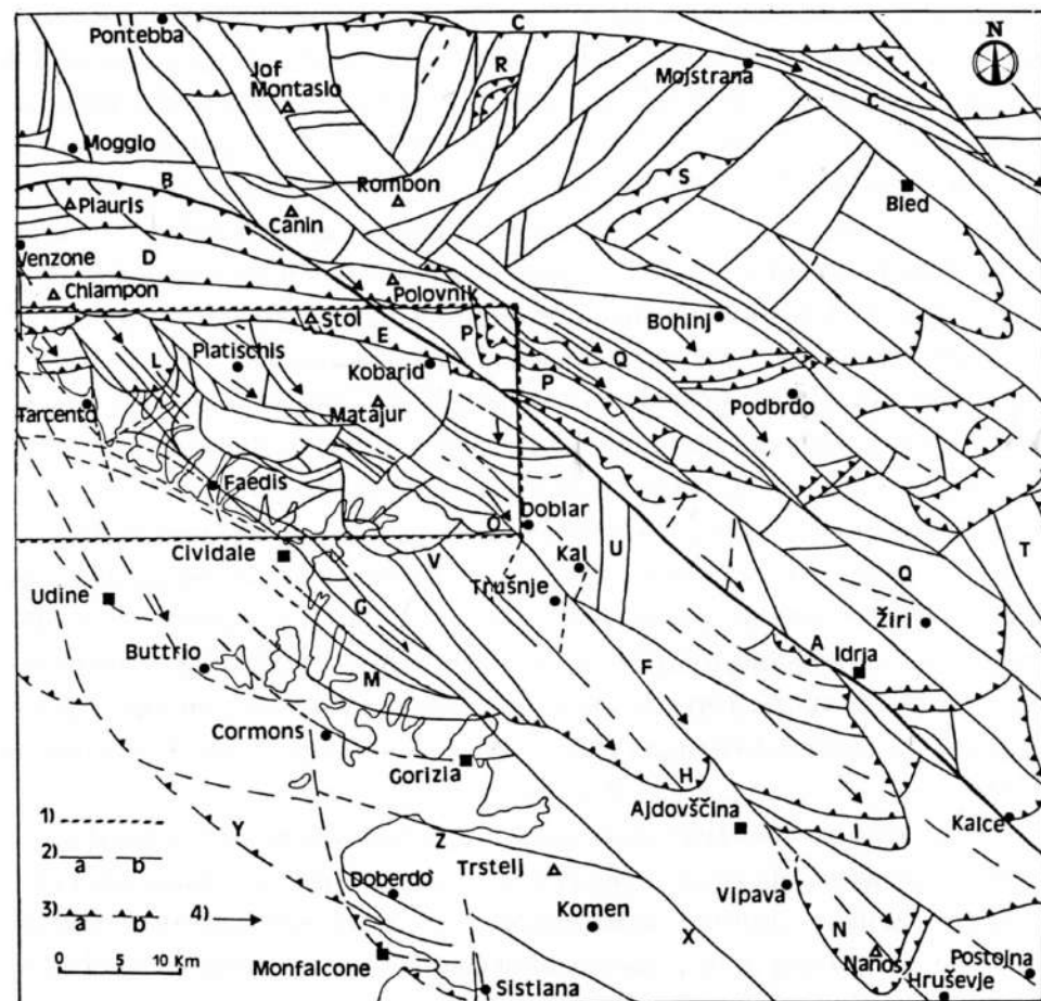
Tav. I - Lineamenti tettonici dell'area di confine italo-iugoslavo. 1. Limiti dell'area di tav. f.t.. 2. Faglie: a) certe; b) presunte o coperte. 3. Sovrascorrimenti: a) certi; b) presunti o coperti. 4. Direzione dei movimenti.
