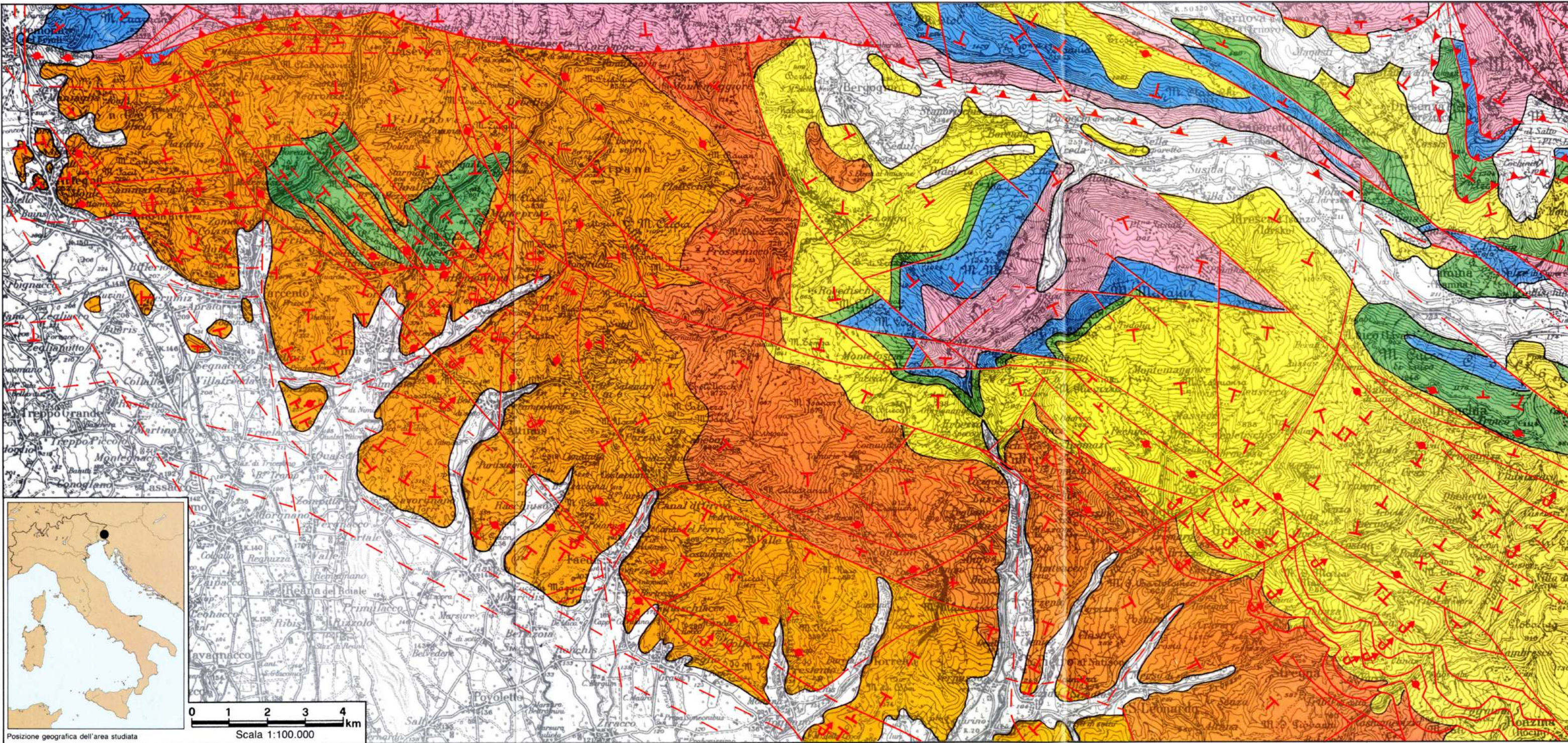
Tavola fuori testo - Schema geologico delle Prealpi Giulie meridionali. - Geologic map of the Southern Julian Prealps.
