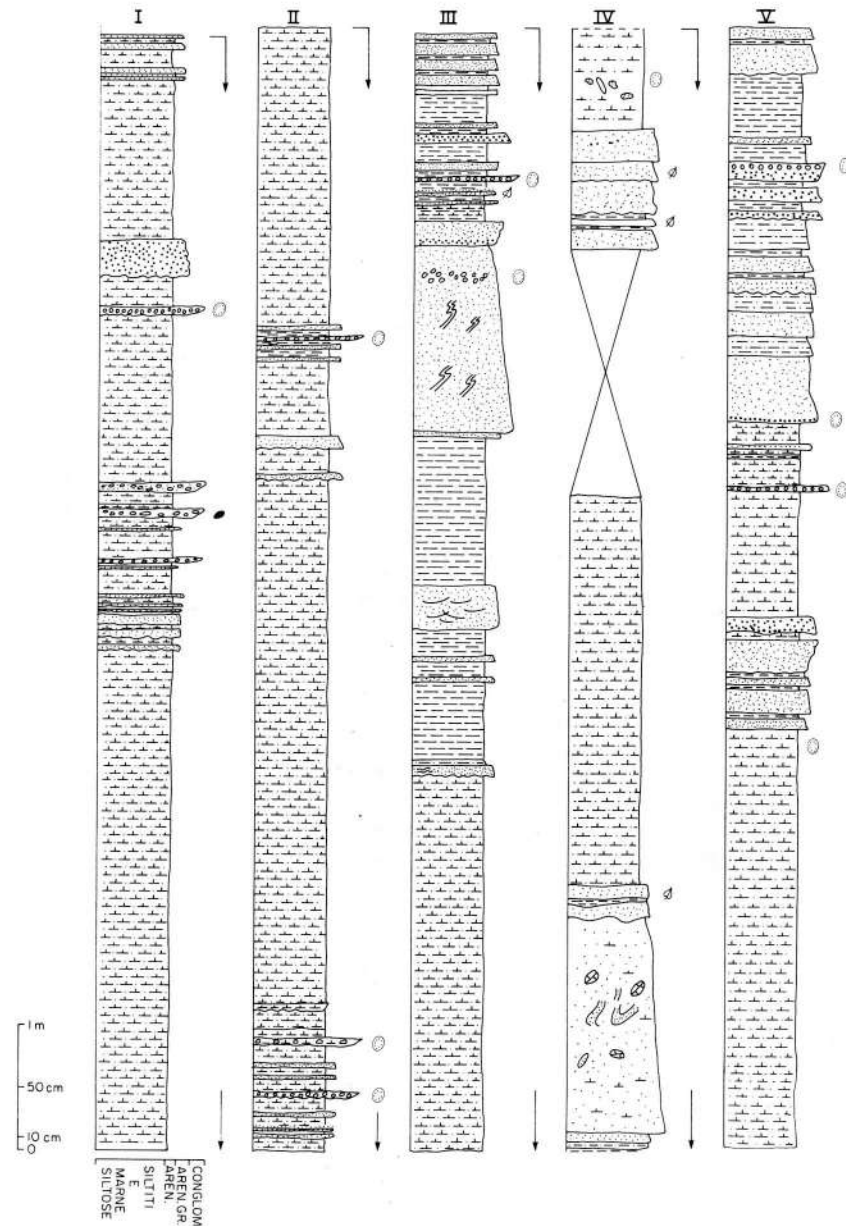
Fig. 9 - Log litologico-sedimentologico della successione Abbazia di Rosazzo. Per i simboli confronta fig. 10.
