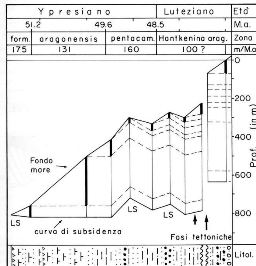
Fig. 14 - Geohistory diagram dei depositi terrigeni eocenici dei colli di Cormons, Rosazzo e Rocca Bernarda. - Geohistory diagram of the eocene clastic deposits of the hills of Cormons, Rosazzo and Rocca Bernarda.
