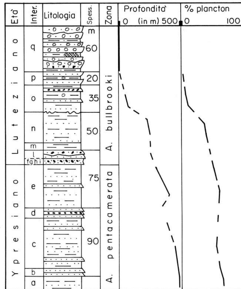
Fig. 4 - Successione stratigrafica dei colli di Cormons. A destra sono schematizzate le variazioni batimetriche e le percentuali dei foraminiferi planctonici. - Stratigraphic sequence of the hills of Cormons. On the right, the bathymetric changes and the planktonic Foraminifera percentages are sketched.
