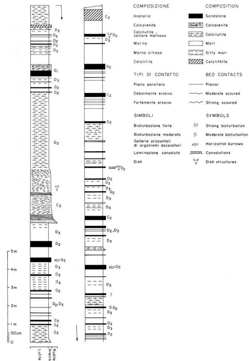
Fig. 8 - Log litologico-sedimentologico della successione C. Nussi (Ipplis). Facies torbiditiche secondo lo schema di MUTTI & RICCI LUCCHI (1975).
