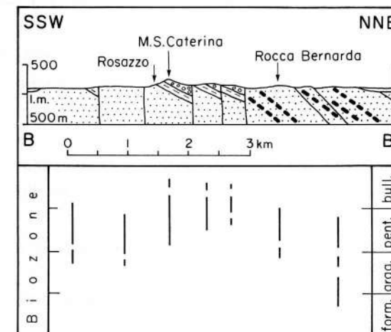
Fig. 7 - Sezione geologica schematica dei colli di Rosazzo e Rocca Bernarda. Traccia della sezione e legenda in fig. 5. In basso, biozone individuate negli spezzoni di successione esaminati. - Cross section along the hills of Rosazzo and Rocca Bernarda. Geological cross section track and text in fig. 5. Below, biozones singled out in the examined parts of the sequence.
