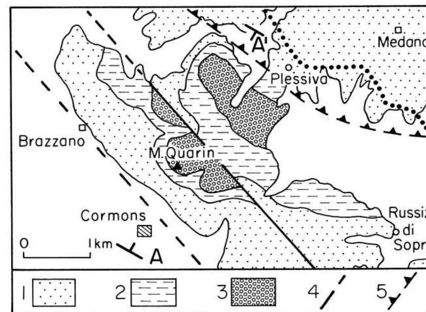
Fig. 2 - Schema di distribuzione delle associazioni di facies dei Colli di Cormons. 1) Torbiditi epibatiali argilloso-arenacee e arenaceo-argillose, con banchi di arenarie amalgamate. Ypresiano-Luteziano basale. 2) Argille siltose e siltiti, talora ciottolose, con frequenti intercalazioni arenacee. Prodelta. Luteziano. 3) Arenarie, siltiti, arenarie conglomeratiche, conglomerati. Fronte e piana deltizia. Luteziano. 4) Faglie subverticali. 5) Sovrascorrimiento. - Distribution map of the main facies associations of the hills of Cormons. 1) Clayey sandy and sandy clayey epibathyal turbidites interbedded with amalgamated thick beds of sandstone. Ypresian-Early Lutetian. 2) Silty clays and siltites, pebbly at times, with several sandy interbeddings. Prodelta. Lutetian. 3) Sandstones, siltites, conglomeratic sandstones, conglomerates. Front and deltaic plain. Lutetian. 4) Subvertical faults. 5) Overthrust.
