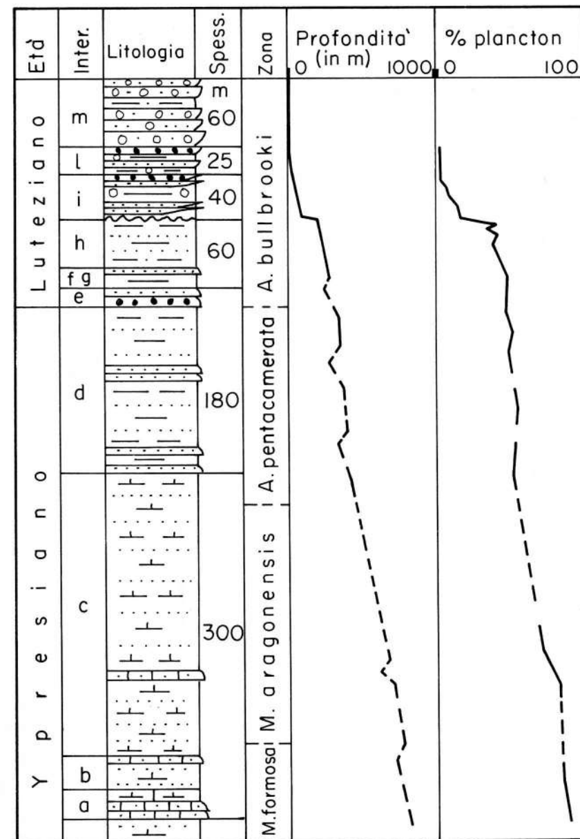
Fig. 5 - Successione stratigrafica dei colli di Rosazzo e Rocca Bernarda. A destra sono schematizzate le variazioni batimetriche e le percentuali di foraminiferi planctonici. - Stratigraphic sequence of the hills of Rosazzo and Rocca Bernarda. On the right, the bathymetric changes and the planktonic Foraminifera percentages are sketched.
