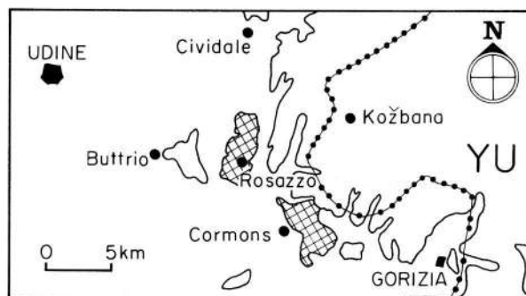
Fig. 1 - Carta indice. In retino è rappresentata l'area esaminata. - Index map. The area under examination is sketched by nets.
