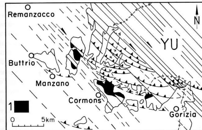
Fig. 12 - Schema tettonico del Collio. 1) Affioramenti di depositi deltizi luteziani. - Tectonic sketch of the Collio region. 1) Outcrops of the lutetian deltaic deposits.
