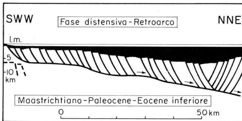
Fig. 15 - Ipotesi paleotettoniche riguardanti l'area di confine italo-ugoslava tra Rosazzo ed il M. Mangart durante il Maastrichtiano-Paleocene-Eocene inferiore (in basso) e l'Eocene medio (in alto). In nero sono rappresentati i depositi terrigeni maastrichtiano-paleocenico-eocenici.
