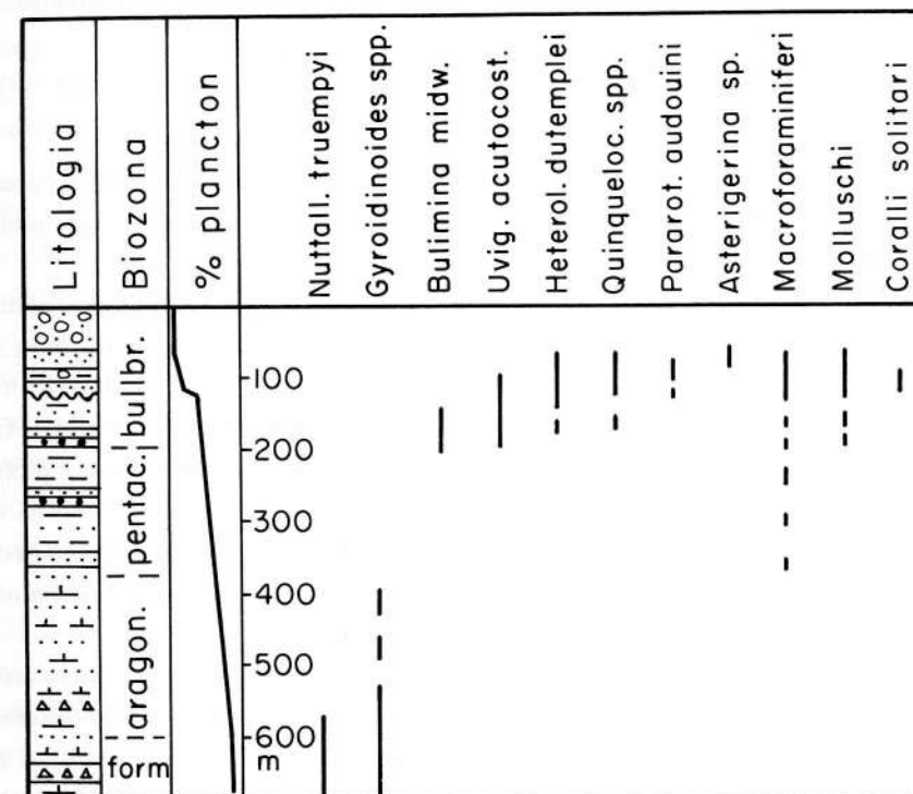
Fig. 11 - Successione stratigrafica dei colli di Rosazzo e Rocca Bernarda con distribuzione di alcune forme di foraminiferi bentonici e macrofossili.
