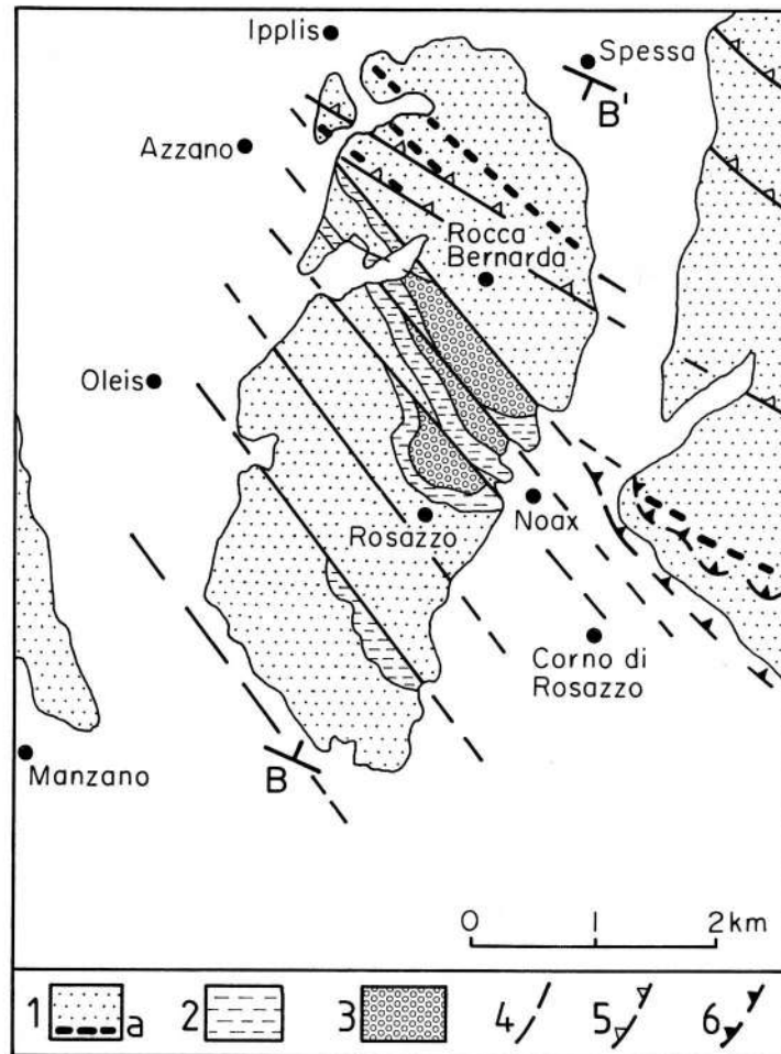
Fig. 6 - Schema di distribuzione delle associazioni di facies dei Colli di Rosazzo e Rocca Bernarda. 1) Torbiditi epibatiali marnoso-arenacee, argilloso-arenacee e arenaceo-argillose; alla base sono presenti banchi carbonatici (a) e calciturbiditi. Ypresiano-Luteziano basale. 2) Argille siltose e siltiti, talora ciottolose, con frequenti intercalazioni arenacee. Prodelta. Luteziano. 3) Arenarie, siltiti, arenarie conglomeratiche, conglomerati. Fronte e piana deltizia. Luteziano. 4) Faglie subverticali. 5) Faglie inverse. 6) Sovrascorrimenti.
