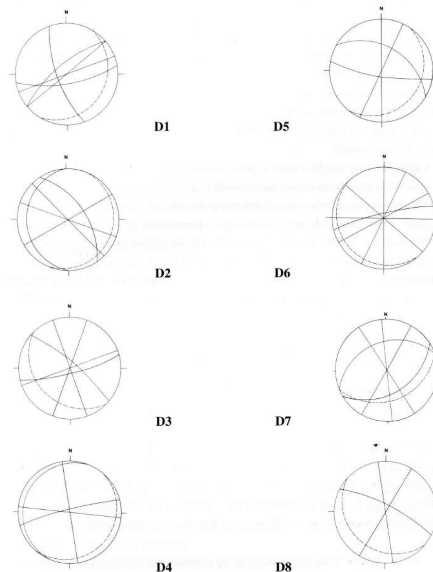
Fig. 2 - Diagrammi strutturali esemplificativi delle diverse situazioni rilevate nell'area studiata. Il grande cerchio a tratteggio rappresenta il piano di strato. La numerazione 1÷8 corrisponde rispettivamente ai numeri 7, 6, 16, 17, 3, 37, 8 e 9 della carta allegata.
