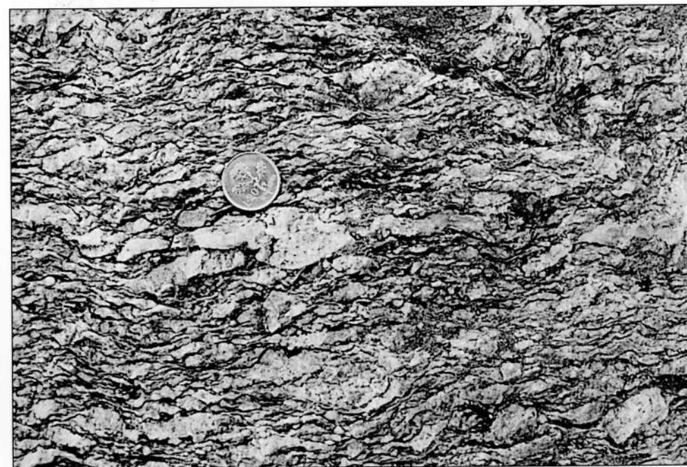
Fig. 4 - Facies tipica degli ortogneiss: si notino i grandi porfirocristalli feldspatici e di quarzo e una piega intrafoliale B_1 (moneta) sradicata su S_{1m} .
