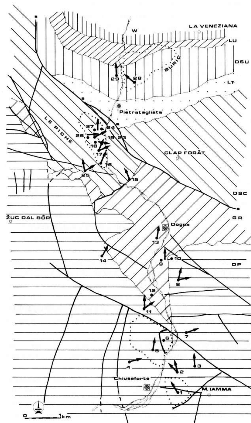
Fig. 1 - Schema geologico con l'ubicazione delle stazioni dell'analisi strutturale e dei fenomeni di D.G.P.V. (circonscritti da linea punteggiata). Le frecce indicano la direzione locale dello stress. DP=Dolomia Principale; GR=Gruppo di Raib; DSC=Dolomia dello Schlem; LT=Formazione di Livinallongo e Torbiditi d'Aupa; DSU=Dolomia del Serla e intercalata Breccia di Ugovizza; LU=Formazione di Lusnizza; W=Formazione di Werfen; i lineamenti più marcati sono le tracce dei principali piani tettonici (s=sovrascorrimento). - Geological sketch on which appear the structural analysis points and the D.S.G.D. areas (in the dotted boundaries). The big lines are the main faults (s=overthrust).
