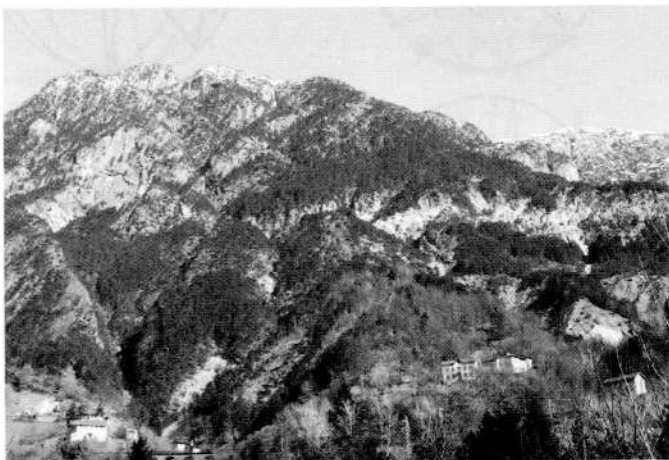
Fig. 3 - Intensa tettonizzazione, con riattivazione, lungo la "linea di Dogna". - High stress fault pattern, reactivated, along the "Dogna fault".
