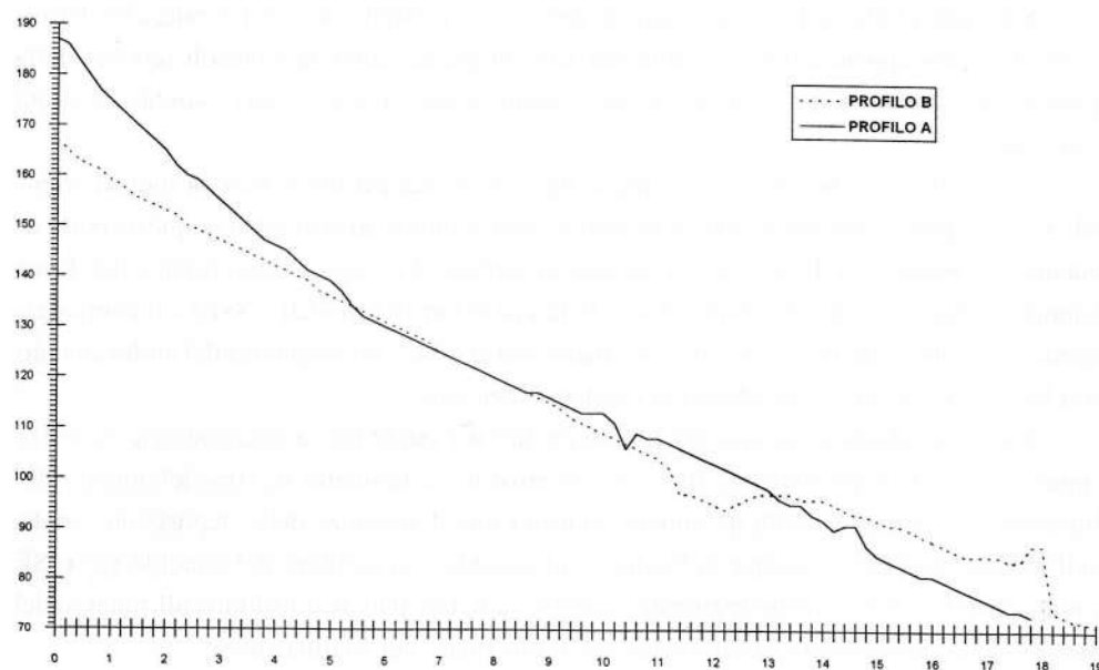
Fig. 7 - Profili longitudinali in destra (linea continua) e in sinistra (tratto) del conoide del Torre. - Longitudinal profiles on the Torre fan, rightside (continuous) and leftside (dotted) of the river bed.
