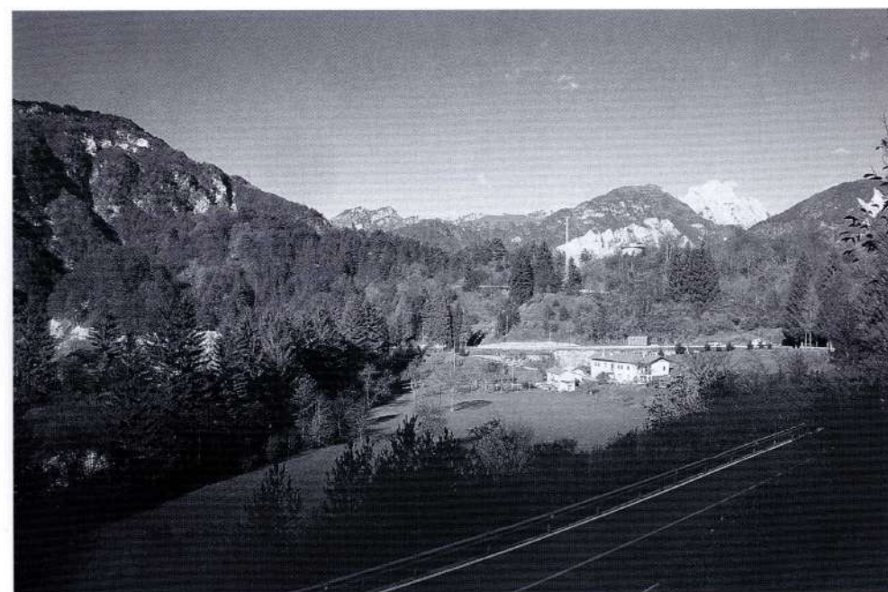
Fig. 2 - Vista da monte della sella sede del paleoalveo del T. Resia. Sulla sinistra l'alveo attuale. - The saddle points out the ancient bed of the Resia River. The actual bed is on the left.
