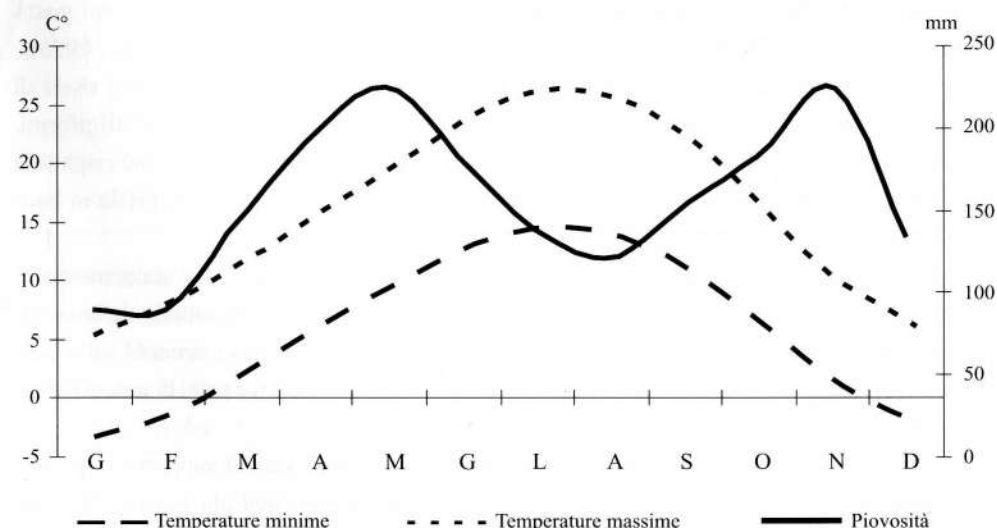
Fig. 2 - Dati pluviometrici (trentennio 1921-1950) e termici (trentennio 1926-1955) relativi alla stazione di Maniago. - Pluviometrical data (years between 1921 and 1950) and temperatures (years between 1926 and 1955) of the station of Maniago.
