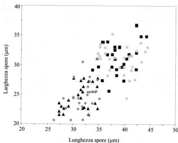
Fig. 1 - Diagramma dei rapporti lunghezza e larghezza delle spore in:
