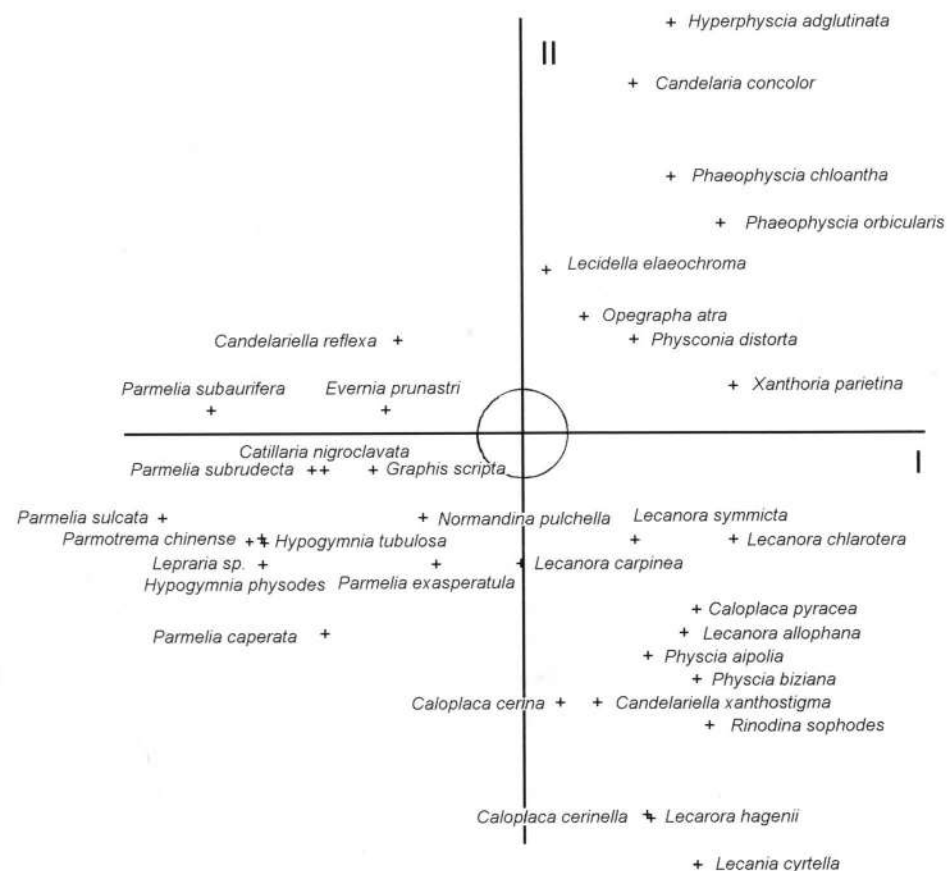
Fig. 7 - Ordinamento delle specie. I punti con alti valori assoluti su entrambe le componenti principali rappresentano le specie caratterizzanti l'ecologia delle comunità licheniche. - Reciprocal ordering of species. The points with higher absolute values on both principal components indicate the most characteristic species of each community.
