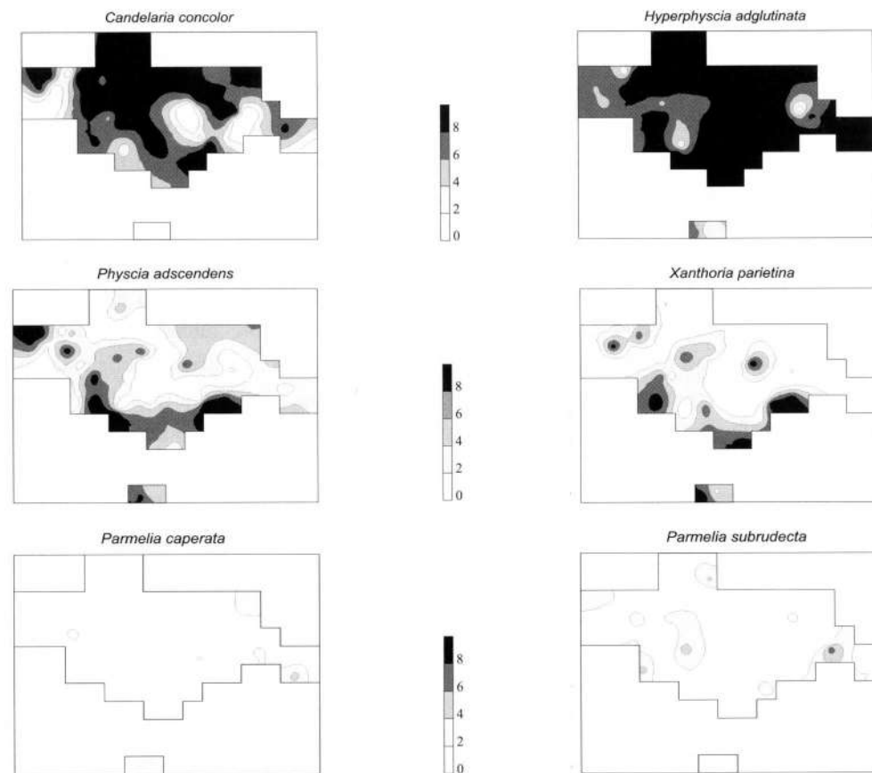
Fig. 8 - Carte di distribuzione nell'area di studio di sei licheni, basate sulla frequenza media nelle 66 stazioni di campionamento.
