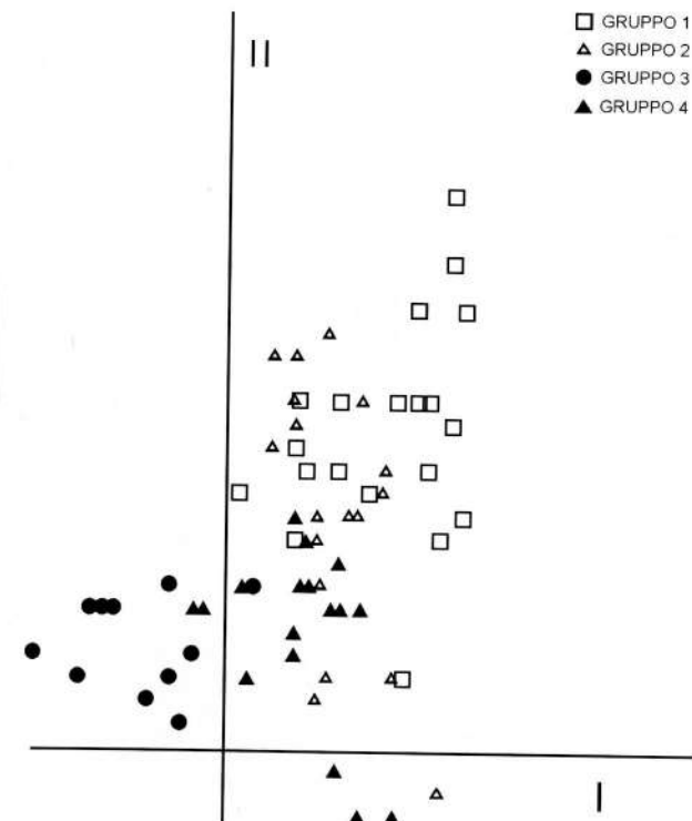
Fig. 6 - Ordinamento delle stazioni di tab. I. I simboli indicano i quattro gruppi evidenziati dalla classificazione di fig. 5, come in legenda. - Reciprocal ordering of stations based on the data of tab. I. The symbols indicate the four main groups obtained by classification (see fig. 5), as in the legend.
