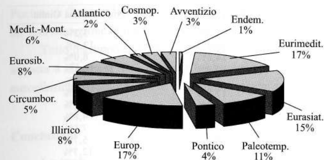
Fig. 9 - Spettro corologico delle specie rilevate nell'area di studio. - Chorological spectrum of species found in the study area.
