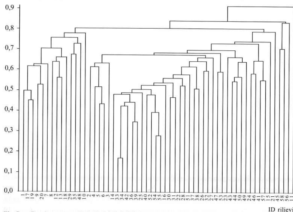
Fig. 7 - Dendrogramma di similarità fra i rilievi. - Similarity dendrogram for relevés.
