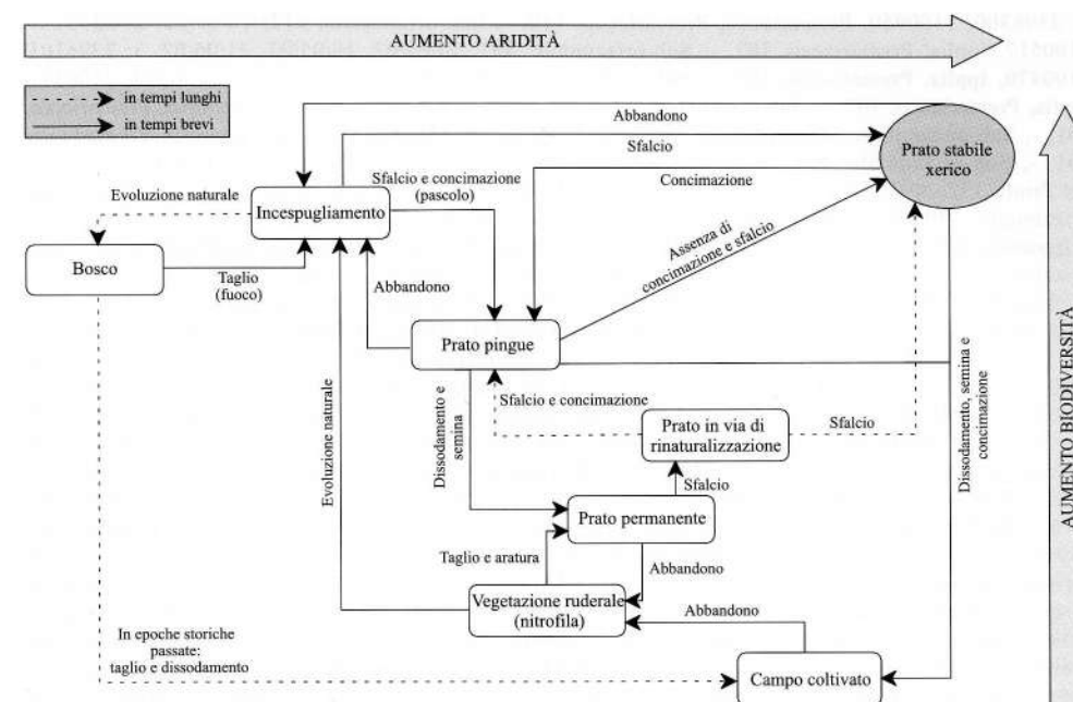
Fig. 10- Schema del dinamismo della vegetazione. - Vegetation dynamism diagram.
