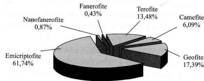
Fig. 8 - Spettro biologico delle specie rilevate nell'area di studio. - Biological spectrum of species found in the study area.
