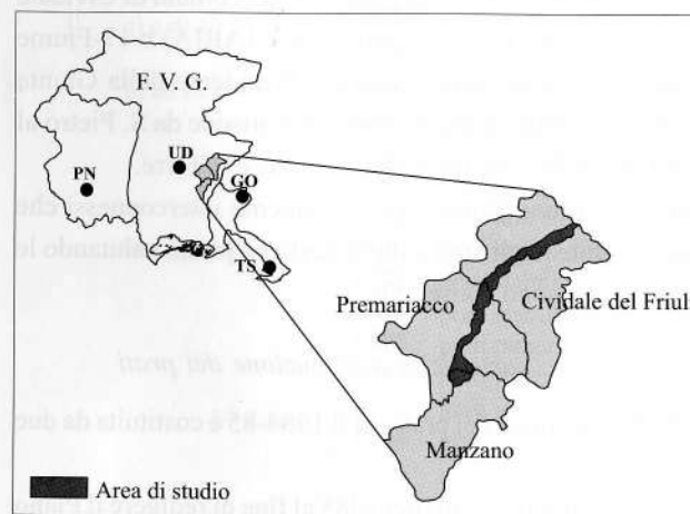
Fig. 1 - Collocazione geografica dell'area di studio. - Map showing the investigated area.
