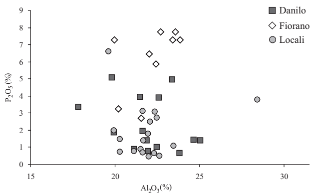
Fig. 16 - Diagramma P_2O_5 vs Al_2O_3 in accordo con la suddivisione culturale-tipologica dei campioni. - P_2O_5 vs Al_2O_3 diagram according to cultural difference of samples.
