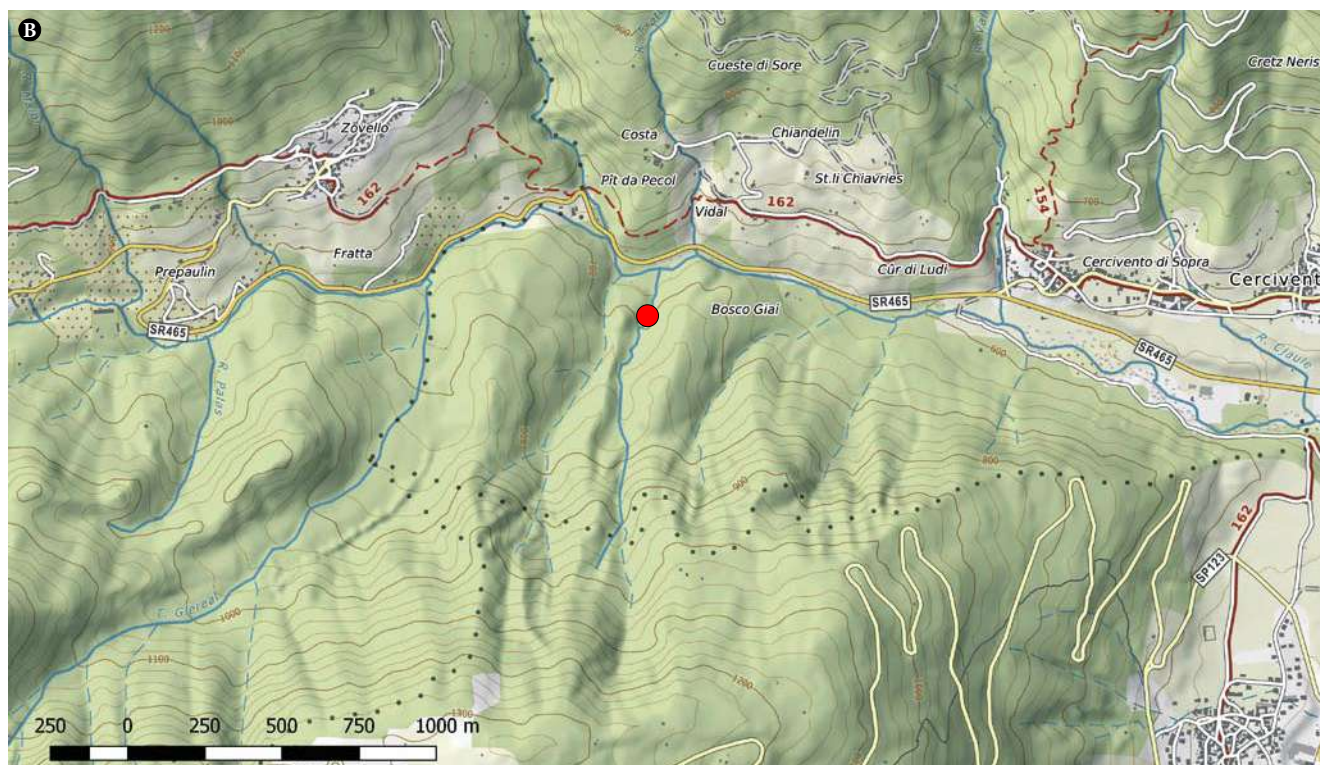
Fig. 1 - A: carta geologica semplificata del settore centrale Carnico (da SELL 1963, mod.; Pm1 = Arenaria di Val Gardena) con le aree del Rio Spinal da Ciare (1) e del Rio Minischitte (2). B: mappa dell'affioramento del Rio Spinal da Ciare (Googlestreet maps). - A: Simplified geological map of the Central Carnic sector (from SELL 1963, mod.; Pm1 = Val Gardena Sandstone) with the areas of Rio Spinal da Ciare (1) and Rio Minischitte (2). B: map of the outcrop of the Rio Spinal da Ciare (Googlestreet maps).
