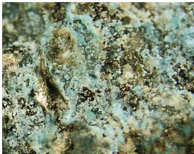
Fig. 10- Arsenolite (cristallini bianchi) e solfoarseniuro di Cu (30x). - Arsenolite (small white crystals) and Cu solfoarseniure (30x).
