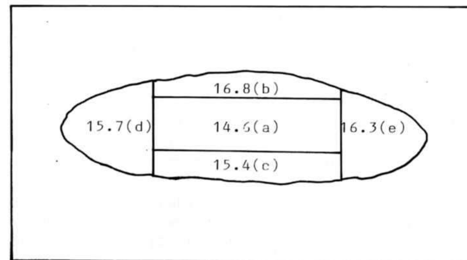
Fig. 1 - Variazione del contenuto in B (ppm) con la posizione nella indocinite Tek 7. Ingrandimento 2X. - Variation of B content (ppm) within the indocinite Tek 7. Enlargement 2X.
