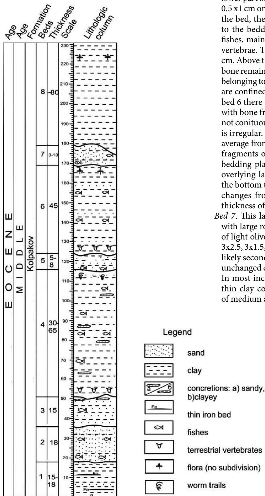
Fig. 9 - Stratigraphic column of the Shynzhily section (drawn by P.E. Pirogova). - Colonna stratigrafica schematica della sezione Shynzhily (disegno di P.E. Pirogova).
