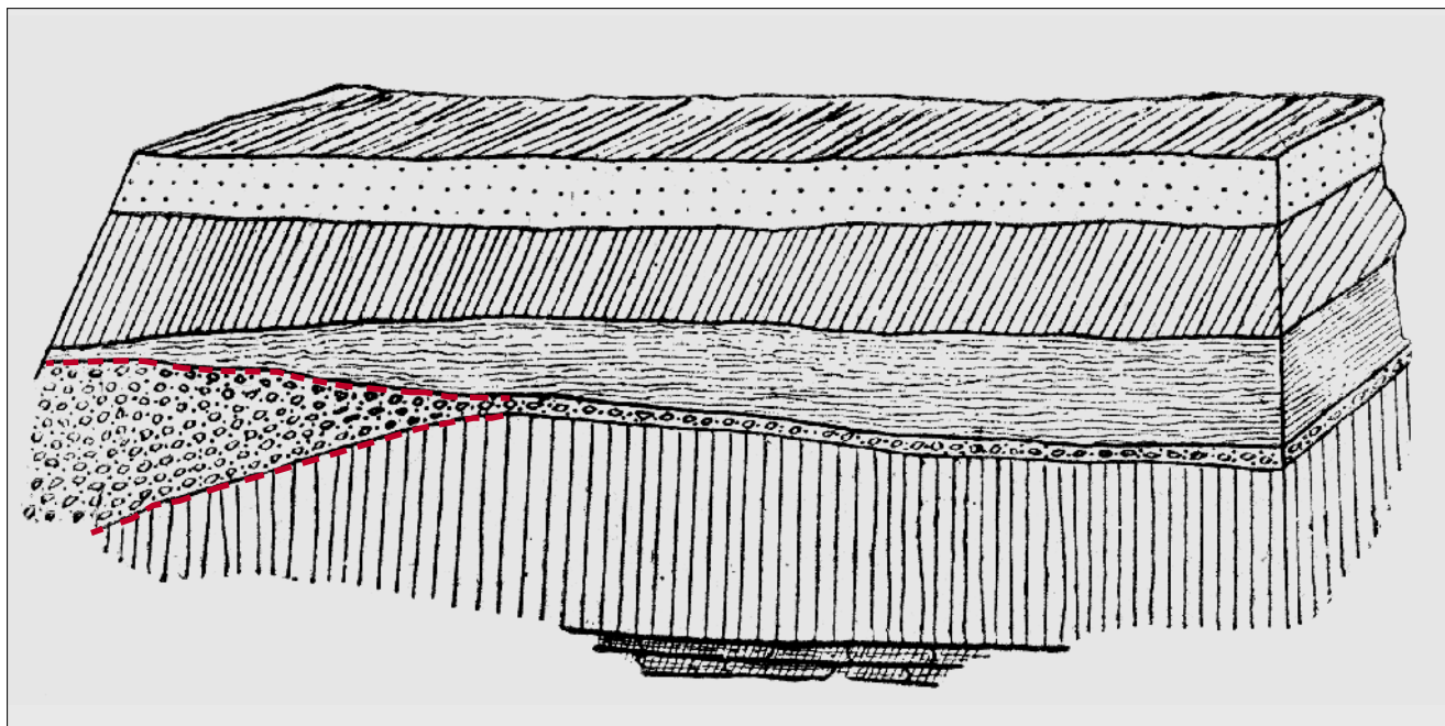
Fig. 15- Sezione trasversale (N-S) tracciata lungo la linea divisoria tra il settore (A) e i sub-settori d-e in (B) (da Feruglio 1921: 8, fig. 3): l'US5 (evidenziata in rosso) aumenta sensibilmente la propria potenza da N a S. - Cross section (NS) drawn along the dividing line between sector (A) and sub-sectors d-e in (B) (from Feruglio 1921: 8, fig. 3): the US5 (highlighted in red) significantly increases its power from N to S.
