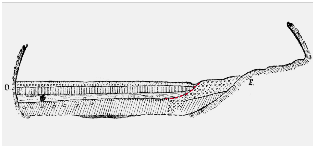
Fig. 12- Sezione trasversale (E-W) della cavità tracciata lungo la linea divisoria tra i sub-settori a-b in (A), d-e in (B) e f-k in (C) con indicazione delle due sequenze stratigrafiche rinvenute. In rosso viene indicata la possibile presenza di un'originaria interfaccia negativa (rielab. da FERUGLIO 1921: 9, fig. 4).
