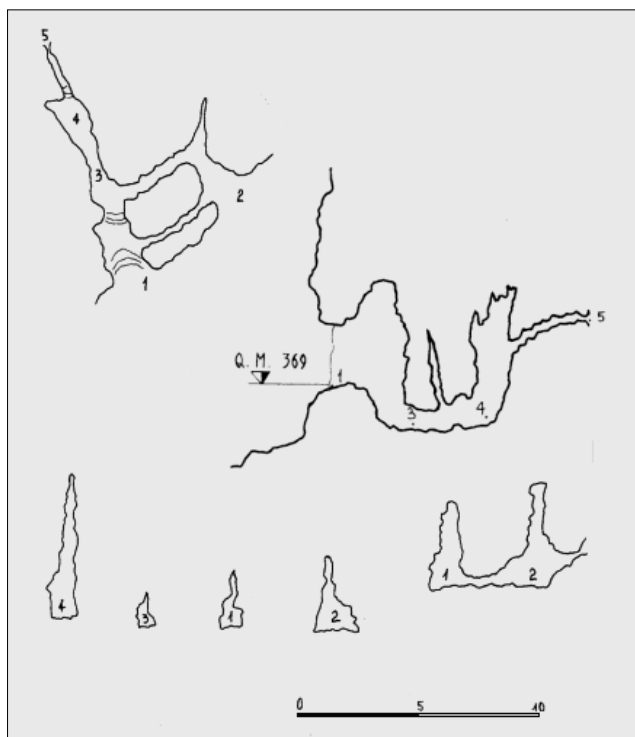
Fig. 2 - Rilievo della galleria principale della Ta pot Figouzo (pianta e sezione) eseguito il 18-08-1957 dal CSIF. - The relief of principal cave of Ta pot Figouzo (plan and section) by the CSIF (18-08-1957).
