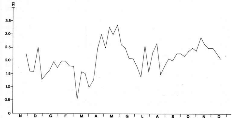
Fig. 5 - Andamento dell'indice di Shannon relativo ai Cladoceri dal novembre 1982 al dicembre 1983. - Changes of Shannon's index of Cladocerans from November 1982 up to December 1983.
