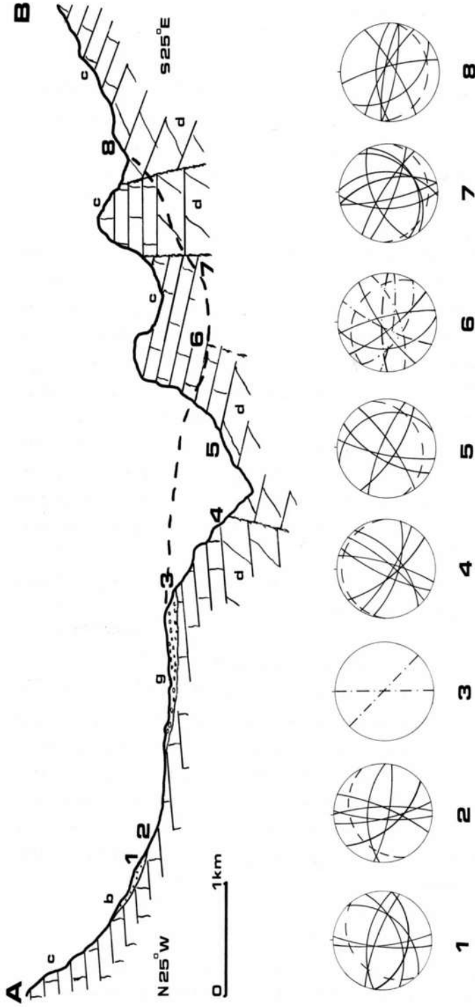
Fig. 2 - Sezione geologica e diagrammi strutturali con la loro ubicazione (1-8). b = breccia di versante; g = morenico e fluvio-glaciale; c = calcari del Dachstein; d = Dolomia Principale. La faglia a tratteggio presso la stazione 6 è la stessa che compare presso il punto 4, essendo la sezione a tratteggio arretrata. Nei diagrammi i grandi cerchi continui sono le discontinuità tettoniche del substrato, quelli a tratto e punto sono in copertura cementata, quelli a tratto sono i giunti di strato. - Geologic profile and location of the structural analysis stations. b = hillside cemented deposits; g = glacial and fluvio-glacial deposits; c = limestones of the Dachstein formation; d = Dolomia Principale. The hatched fault near station 6 is the same near station 4, because the hatched section is upvalley. The continuous great circles are tectonic joints in bedrock, the hatched ones are strata joints and the dot and hatch ones are tectonic joints in conglomerates.
